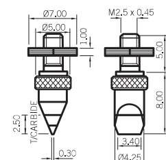
Knife Edge
