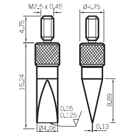
4 x 11mm Knife Edge
