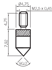
90° Tip
