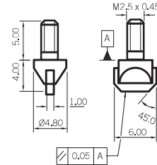
1 x 6mm Blade Edge
